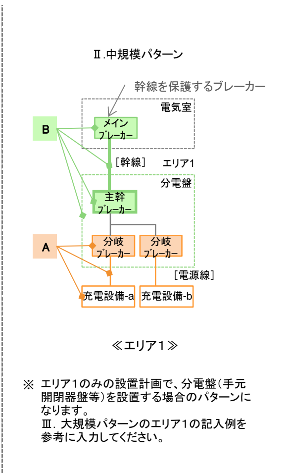
様式4-2：工事申告書(工事内容)の記入例(充電設備を複数基設置する申請の場合)
