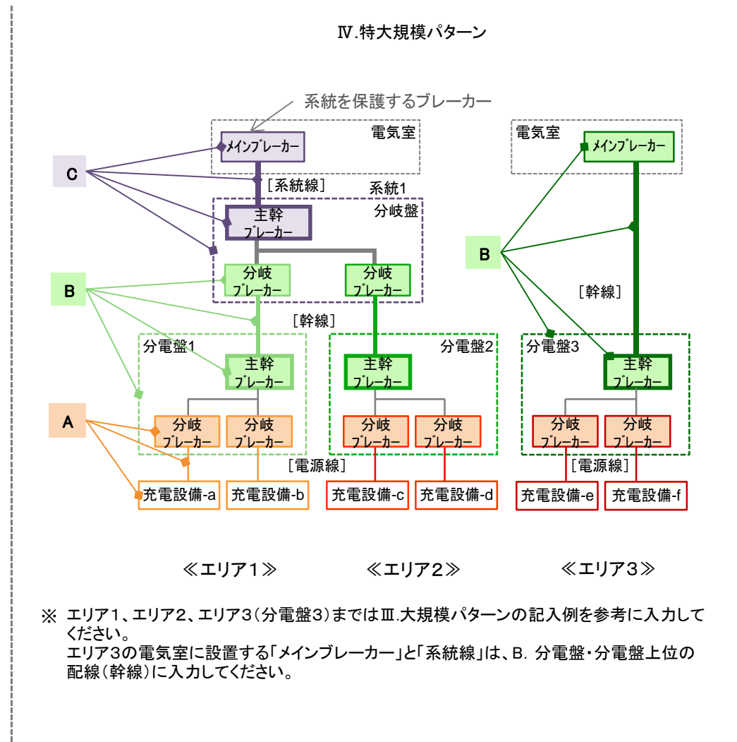
申告する工事の仕様および工法の入力方法についての説明
