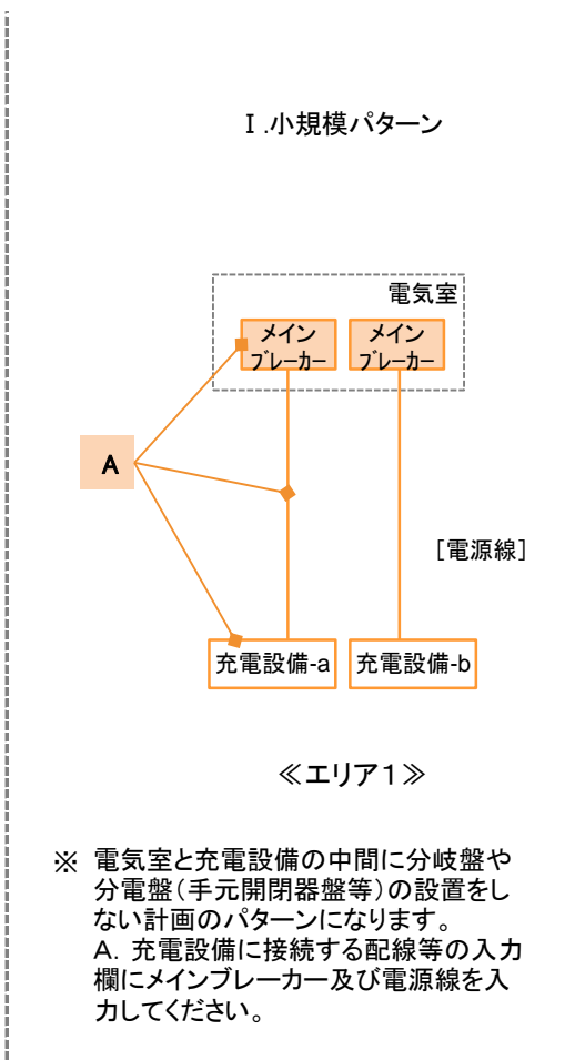
様式4-2：工事申告書(工事内容)の記入例(充電設備を複数基設置する申請の場合)
