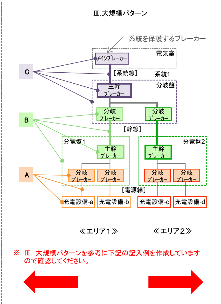
様式4-2：工事申告書(工事内容)の記入例(充電設備を複数基設置する申請の場合)
