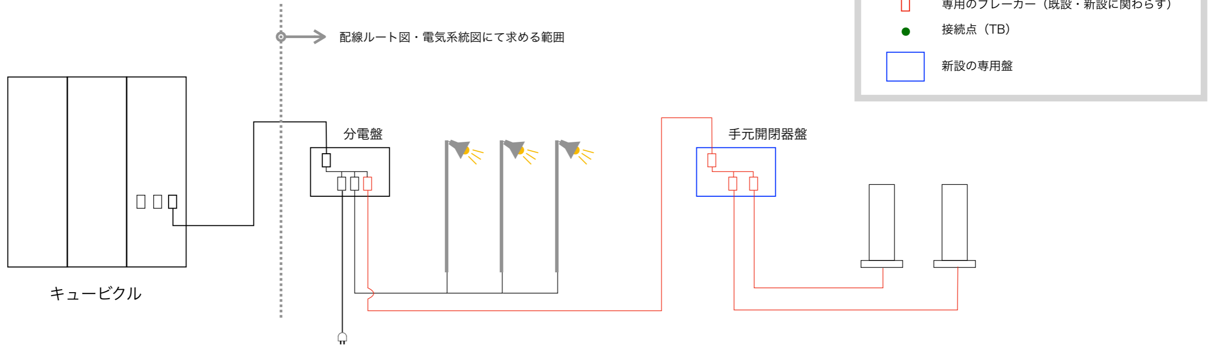
パターン③ 充電設備の専用ではない分電盤と手元開閉器盤
