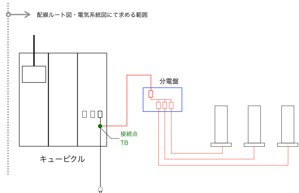
パターン⑤ 充電設備の専用分電盤
