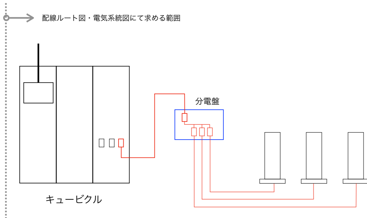
パターン④ 充電設備の専用分電盤
