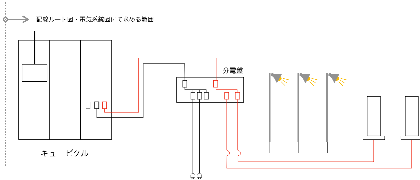
パターン② 充電設備の専用ではない分電盤
