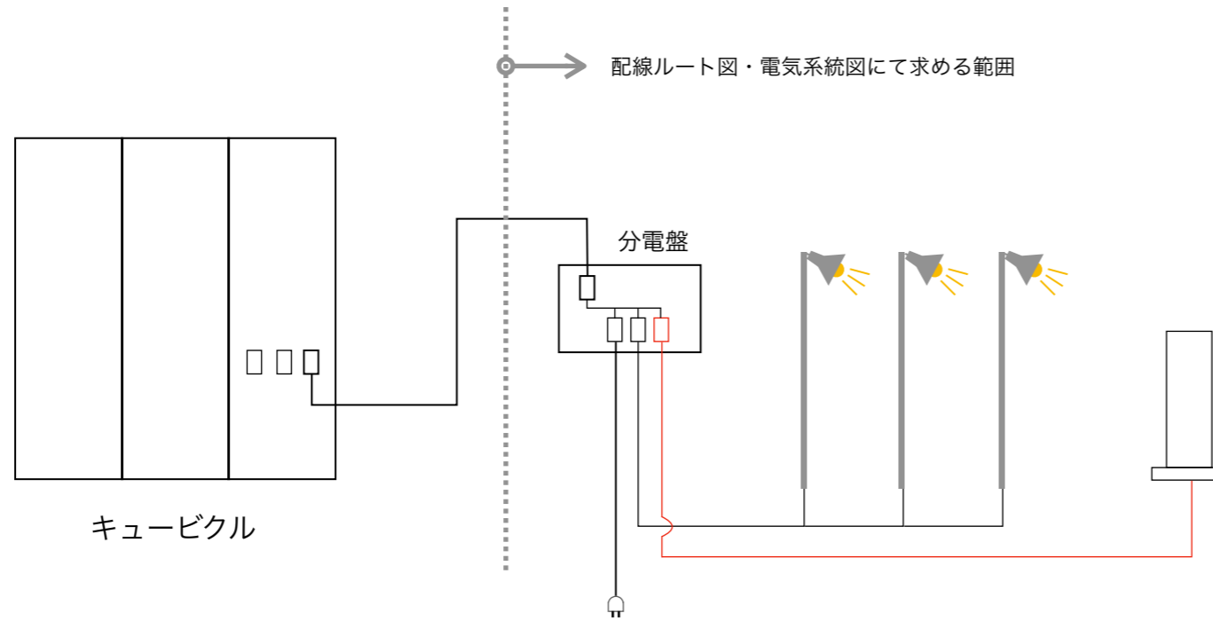
パターン① 充電設備の専用ではない分電盤
